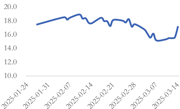
图表 7: VIX 指数
